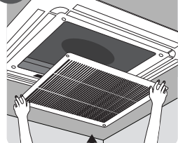
Монтаж лицевой панели
