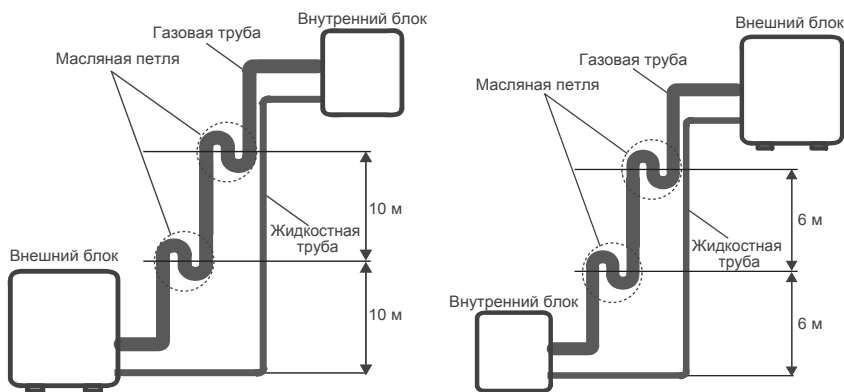
1. Внутренний блок установлен выше наружного блока 2. Внешний блок установлен выше внутреннего блока
