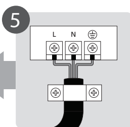
Подключение питающего кабеля
