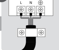
Подключение питающего кабеля
